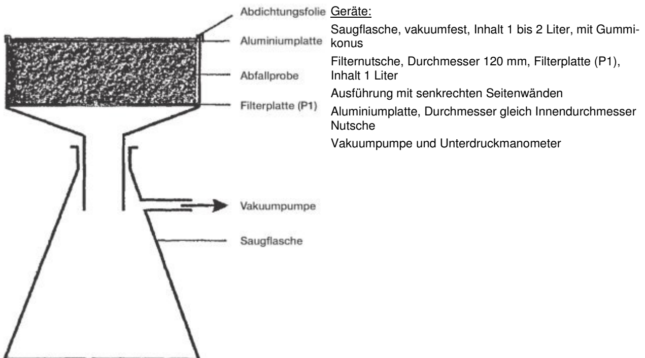
Bild 1: Apparatur zur Einstellung des Wassergehaltes
