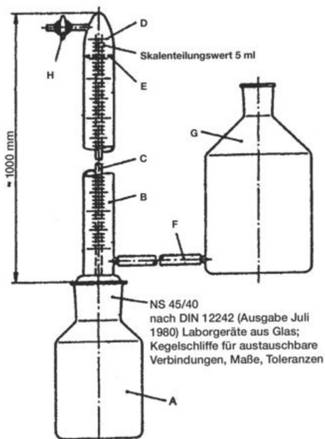
Bild 2: Versuchsapparatur zur Bestimmung des Faulverhaltens von Schlämmen nach DIN 38414-8, Seite 6, Ausgabe Juni 1985
